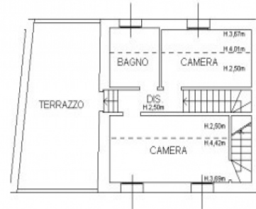
PIANO PRIMO
